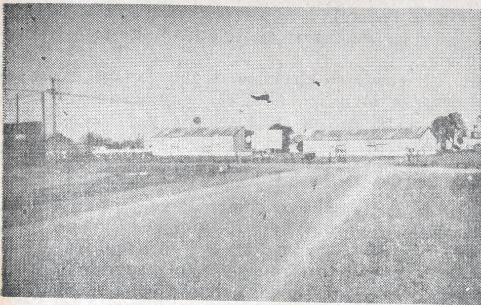
El acceso en la recta hacia la Ruta N° 131 Obra F. Cacik e Hijos
